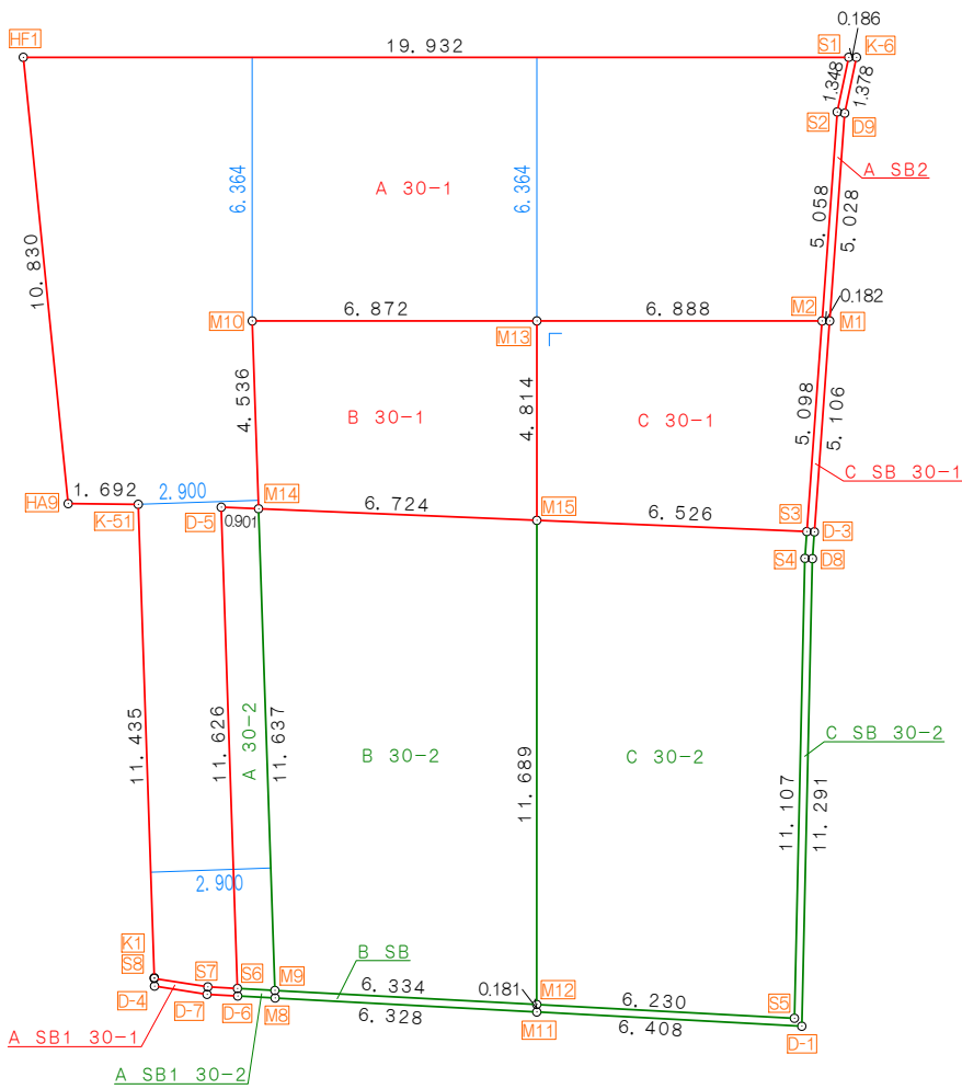
A SB1 30-1ほか 拡大図 1/25
